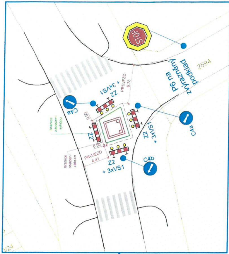
SITUACE M 1:250
